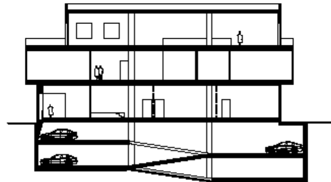
CORTE LONGITUDINAL
